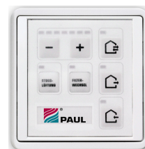
Panel obsługi z 7-stopniową regulacją (Wymiary : 80x80x12 mm) z program komunikacji PEHA,
